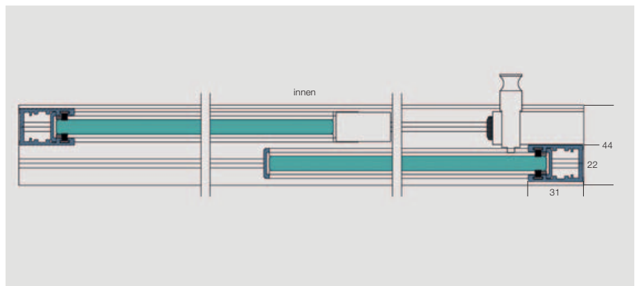
Horizontalschnitt
